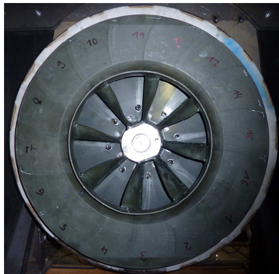
Bild 1: Testrotor eines Heißgasventilatorlaufrades auf dem Prüfstand
